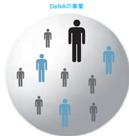
球の表面積
